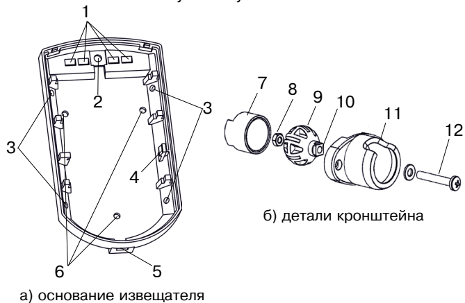
Рисунок 2 – Основание извещателя и кронштейн
