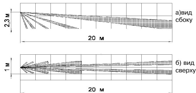
Рисунок 1 – Диаграмма зоны обнаружения
