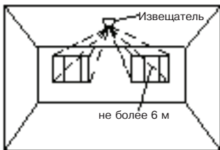
Рис. 26-Установка извещателя на потолок
