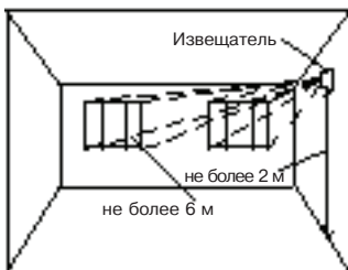
Рис. 28-Установка извещателя на противоположной стене
