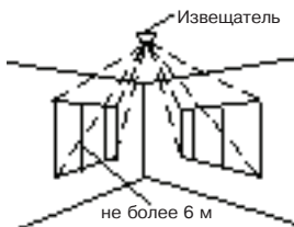
Рис. 27-Установка извещателя на боковой стене
