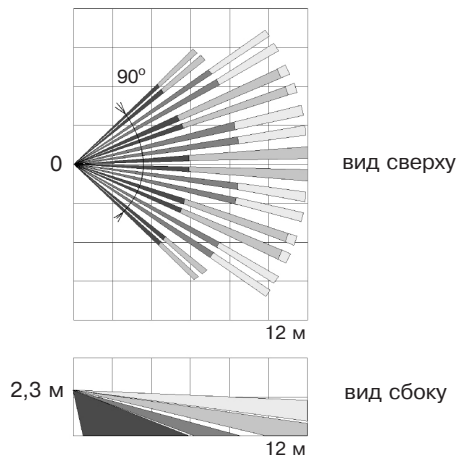
Рисунок 1 – Диаграмма зоны обнаружения известателя «Фотон-12-РК»
