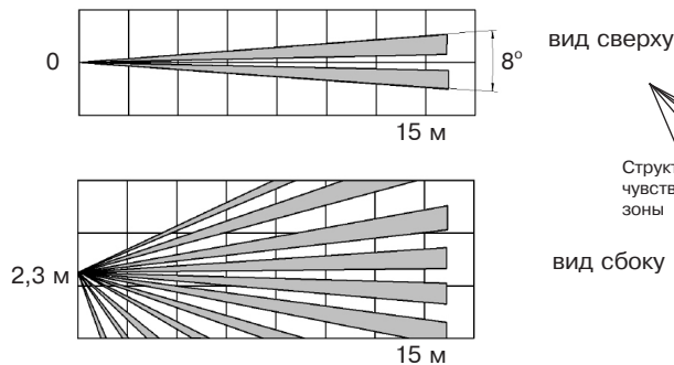
Рисунок 2 – Диаграмма зоны обнаружения известателя «Фотон-12Б-РК»
