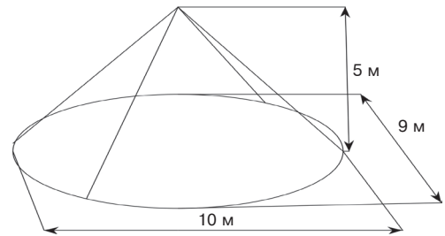
Рисунок 1 – Диаграмма зоны обнаружения
