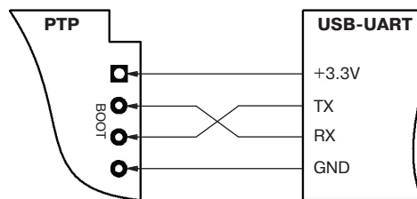
Рисунок 2 – Схема подключения преобразователя
