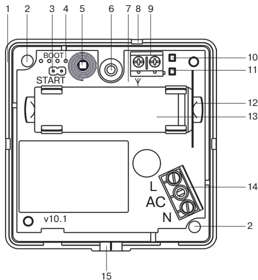
Рисунок 1 – РТР со снятой крышкой
