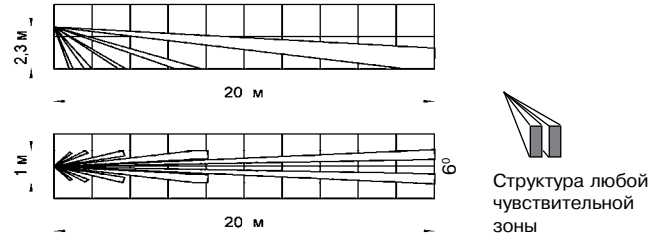
Рисунок 1 – Диаграмма зоны обнаружения
