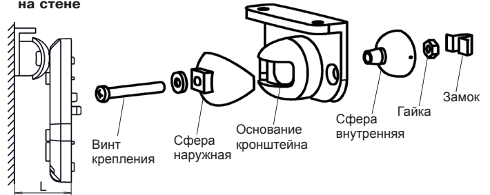
Рисунок 2 – Основание извещателя и кронштейн
