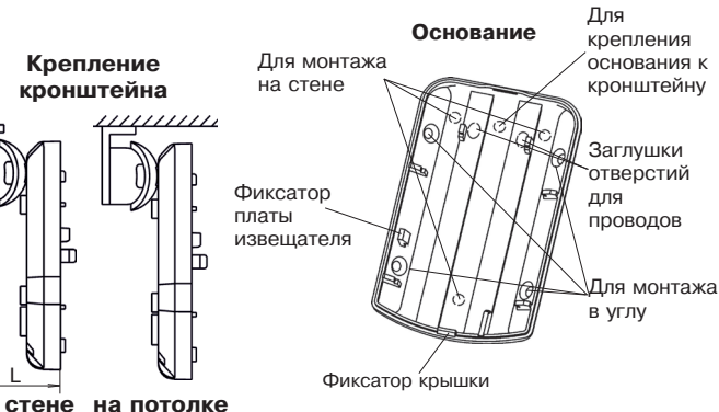
Рисунок 2 – Основание извещателя и кронштейн
