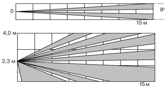
Рисунок 1 – Диаграмма зоны обнаружения
