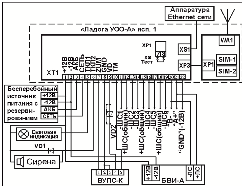
Рисунок А.1 – Схема соединений для проверки УОО после монтажных работ
