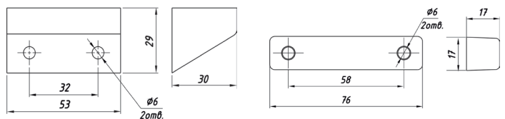
Рисунок 2 – Габаритно-присоединительные размеры
