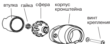
Рисунок 3 – Детали кронштейна
