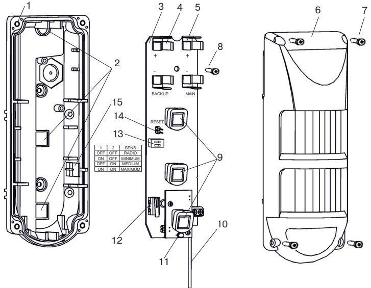
Рисунок 1 – Конструкция «Пирон-8Б-РК»
