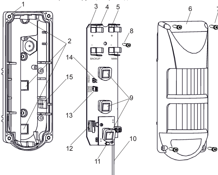
Рисунок 1 – Извещатель
