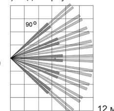
Рисунок 2 – Диаграмма зоны обнаружения
