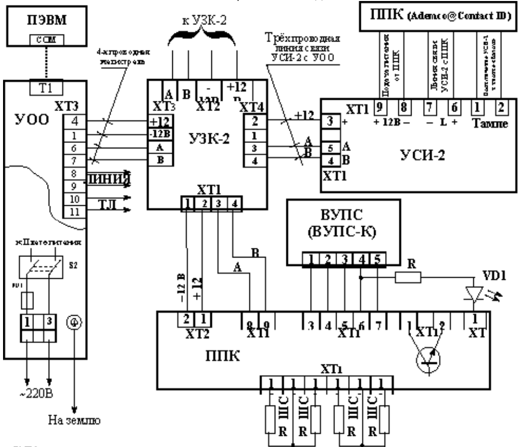
Схема электрических соединений
