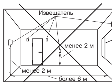
Рисунок 7 – Нерекондуемые места установки извещателя
