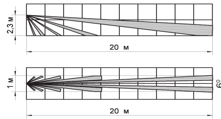
Рисунок 1 – Диаграмма зоны обнаружения
