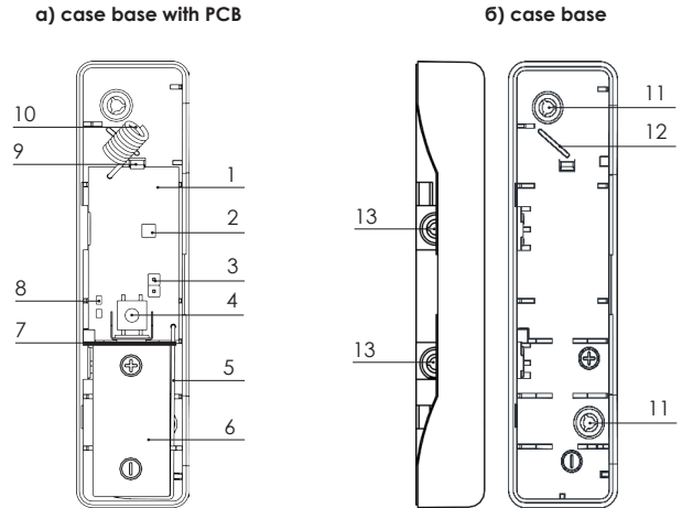
Picture 1 – «Ri-TD-1» detector case
