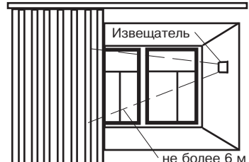
Рисунок 6 – Установка извещателя между стеклом и занавесями (жалюзи)
