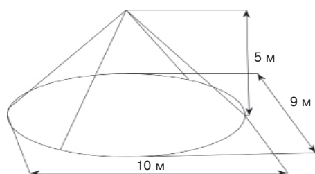
Рисунок 1 – Диаграмма зоны обнаружения
