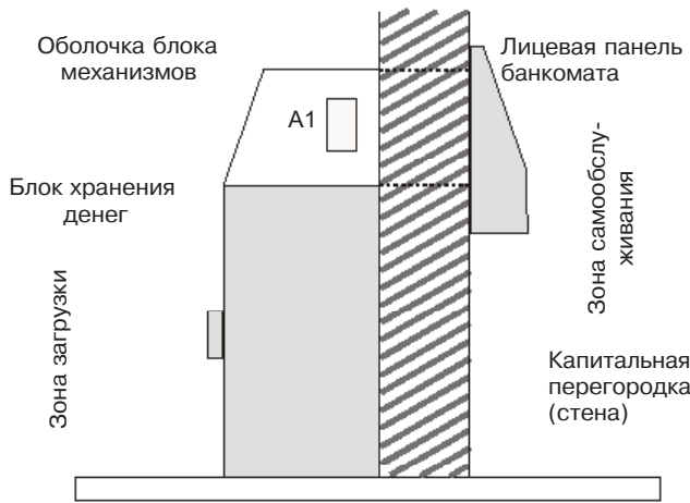
Рисунок 5 – Защита банкомата
