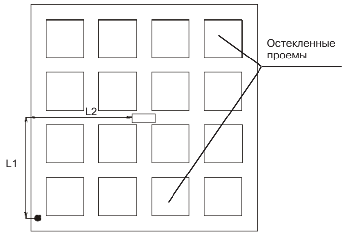
Рисунок 6 – Защита переплета оконной рамы
