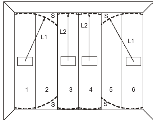
Рисунок 7 – Защита немонолитной конструкции
