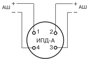
Рисунок 2 – Схема подключения извещателя
