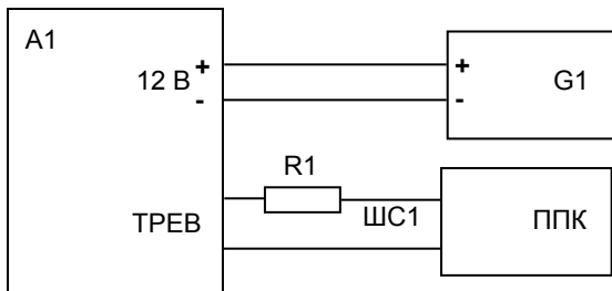
Рисунок 1 – Схема подключения извещателя
