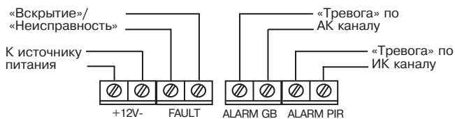
Рисунок 4 – Схема подключения извещателя
